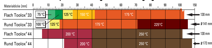
Vorwärmtemperatur bei austenitischem Schweißgut 125 °C ab 20 mm Blechdicke.
